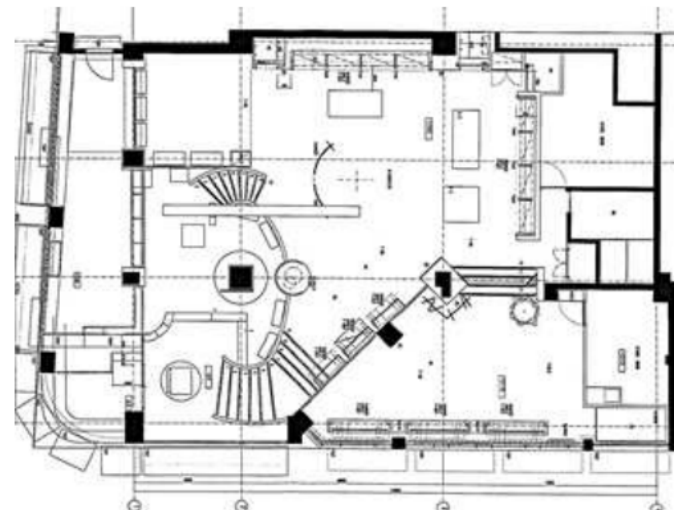
平面図
